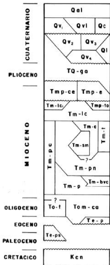
Fig. 2: Columna estratigráfica. Complejo de Nicoya (Ken), Fm. Punta Serrucho (Te-ps), Fm. Parritilla (Te-p), Fm. Caraiques (Tom-ca), Miembro Tranquerillas (To-t), Fm. Punta Carballo (Tm-pc), Fm. Pacacua (Tm-p), Brechas verdes Coyolar (Tm-bvc), Fm. Peña Negra (Tm-pn), Fm. San Miguel (Tm-sm), Fm. Coris (Tm-c), Fm. Turrúcares (Tm-t), Fm. La Cruz (Tm-lc), Depósitos Parálitos de Fm. La Cruz (Tm-lci), Tobitas Ococa (Tm-to), Intrusivo de Escazú (Tm-e), Cornubianitas de Escazú (Tm-ce), Fm. Grifo Alto (TQ-ga), Fm. Lavas intracañón (Qv4), Fm. Depósitos de Avalancha Ardiente (Qv3), Fm. Orotina (Qv2), Fm. Barva (Qv1), Depósitos lacustres (Ql), Calizas deslizadas (Qc), Lahares y cenizas (Qv1), Depósitos aluviales y coluviales recientes (Qal).
